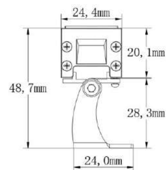
■产品尺寸图
