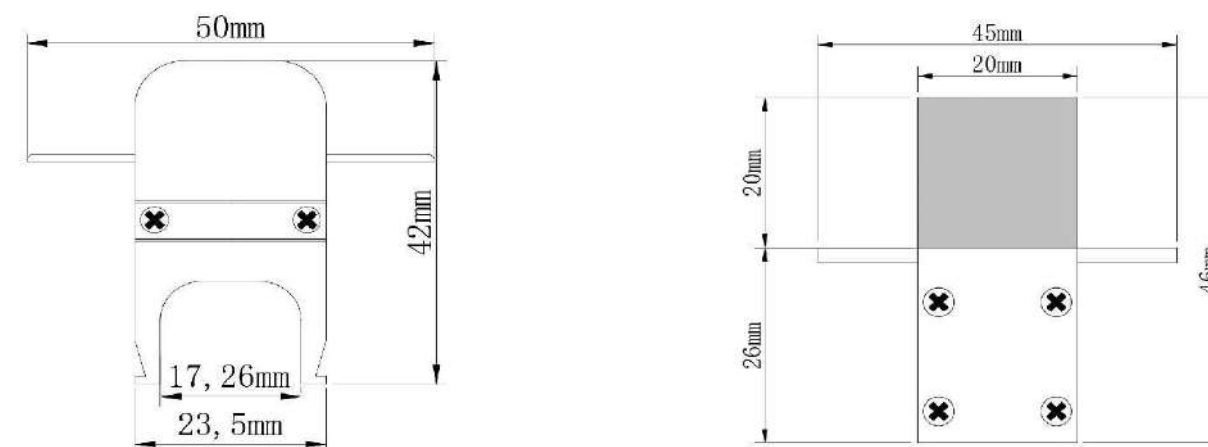
产品尺寸图
