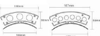
产品尺寸图
