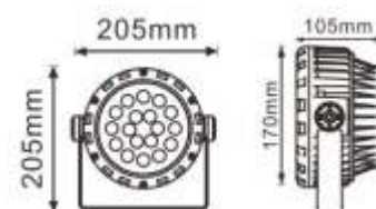
■产品尺寸图
