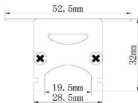
产品尺寸图
