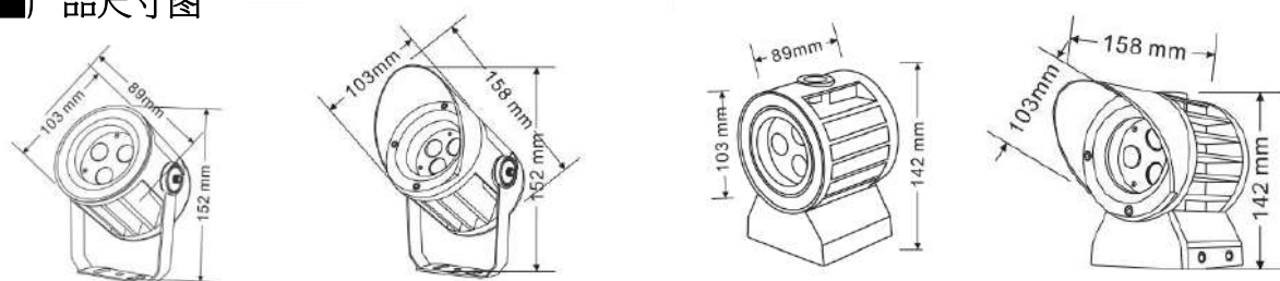
■产品尺寸图
