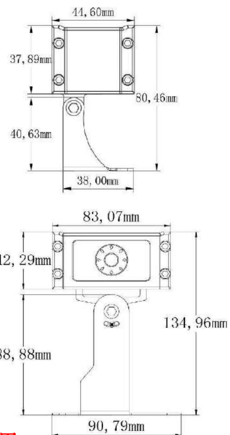
■产品尺寸图
