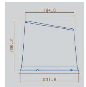
■产品尺寸图
