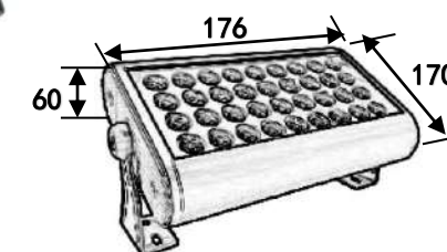
■产品尺寸图
