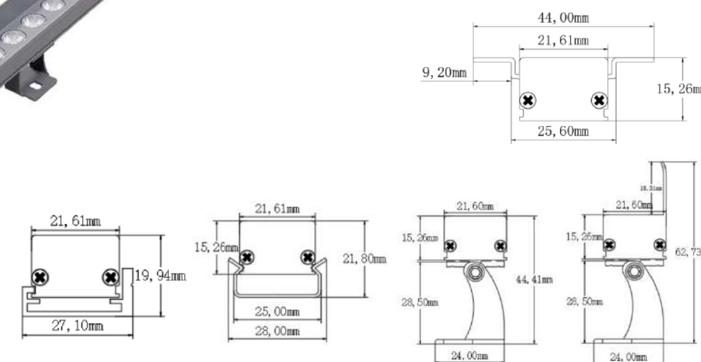
产品尺寸图
