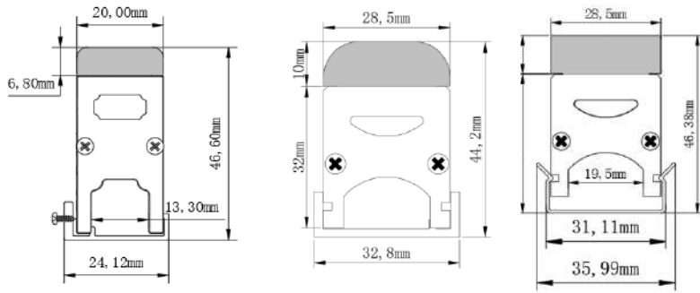
产品尺寸图
