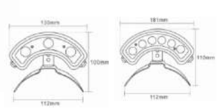
产品尺寸图
