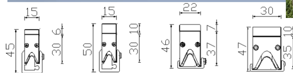
产品尺寸图
