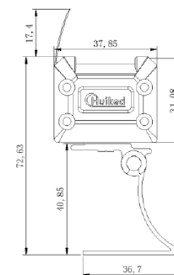
产品尺寸图
