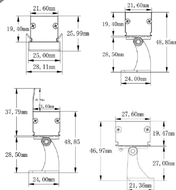
产品尺寸图
