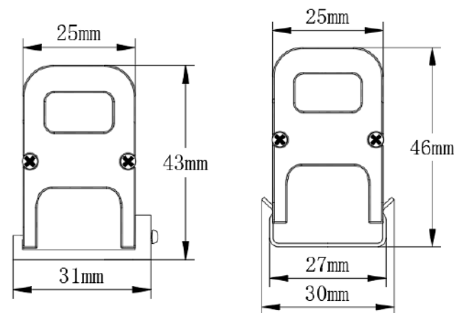
产品尺寸图
