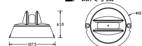
■产品尺寸图
