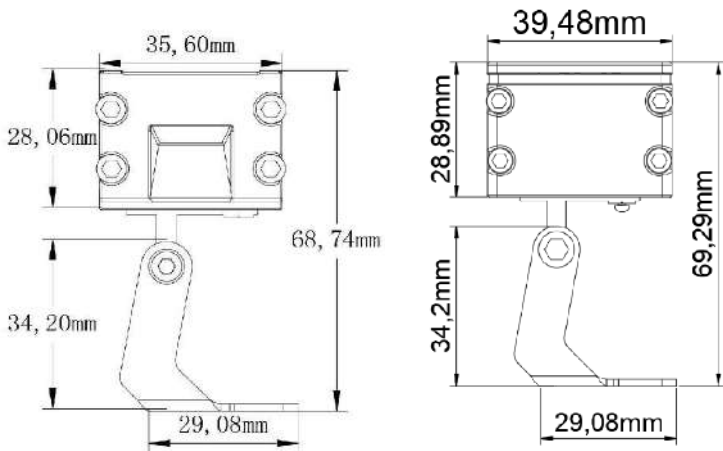
产品尺寸图
