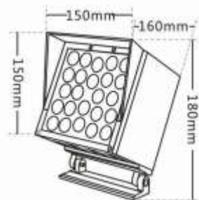
产品尺寸图
