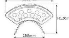
产品尺寸图
