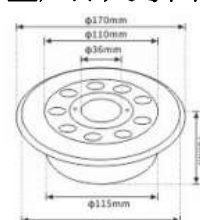
■产品尺寸图
