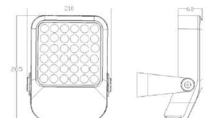
产品尺寸图
