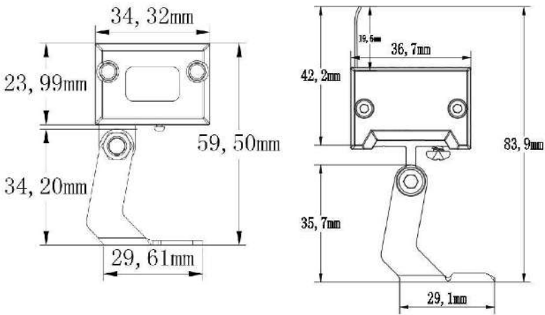
产品尺寸图
