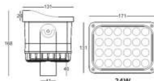
■产品尺寸图
