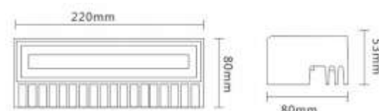
■产品尺寸图
