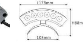
产品尺寸图
