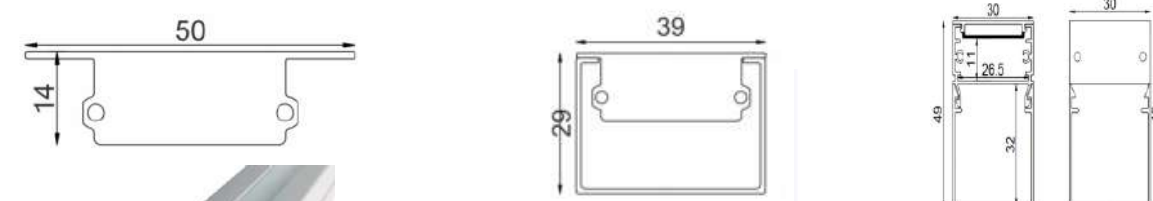
产品尺寸图
