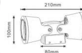
■产品尺寸图
