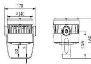
■产品尺寸图
