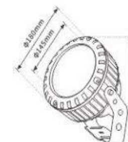
■产品尺寸图
