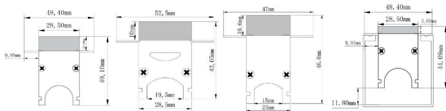
产品尺寸图
