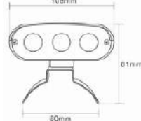
产品尺寸图
