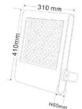
产品尺寸图
