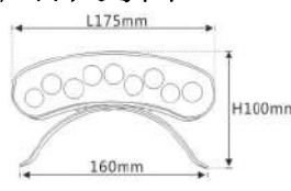
产品尺寸图
