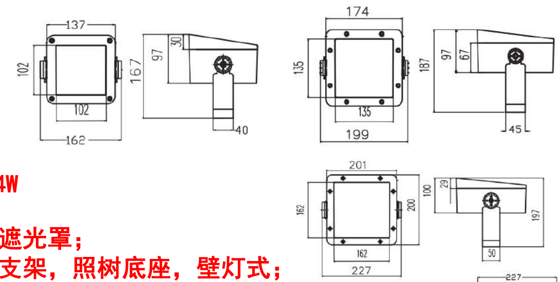
■产品尺寸图
