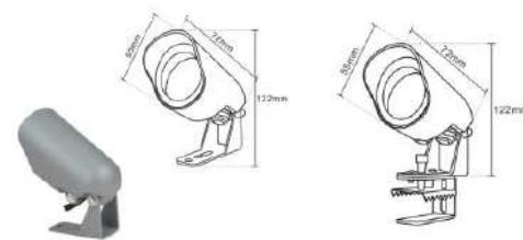
■产品尺寸图
