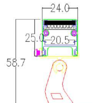
带格栅条
