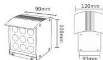
■产品尺寸图
