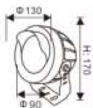
■产品尺寸图
