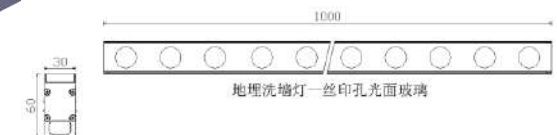
■产品尺寸图
