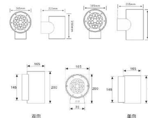
产品尺寸图
