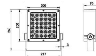
■产品尺寸图
