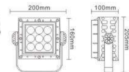
产品尺寸图
