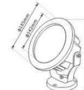
■产品尺寸图
