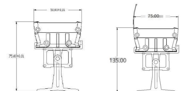
产品尺寸图
