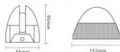
■产品尺寸图
