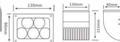
■产品尺寸图
