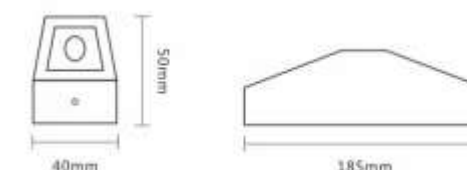
■产品尺寸图
