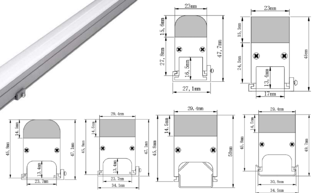
产品尺寸图
