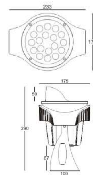
■产品尺寸图
