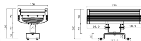
■产品尺寸图
