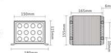
产品尺寸图
