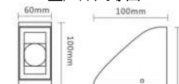
■产品尺寸图
