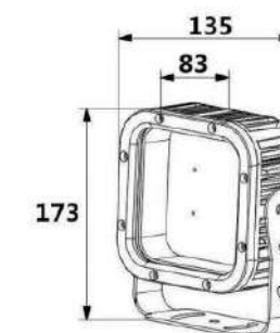
■产品尺寸图
