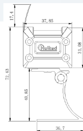
产品尺寸图
