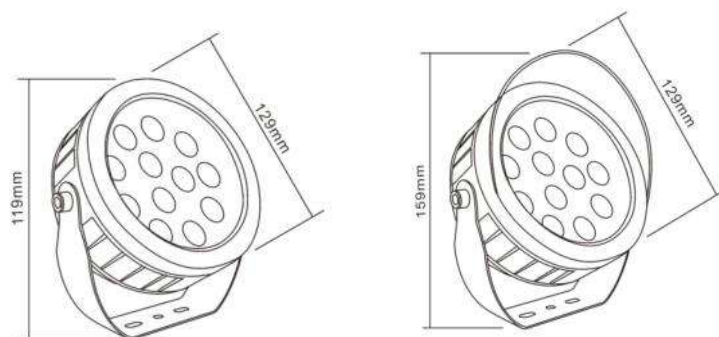
产品尺寸图
