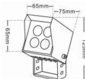
产品尺寸图
