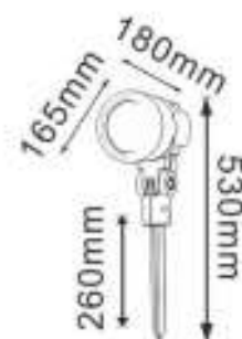
■产品尺寸图
