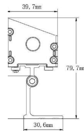
产品尺寸图
