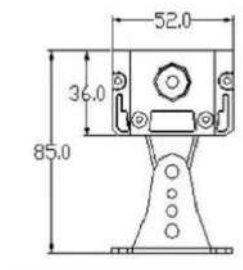
■产品尺寸图
