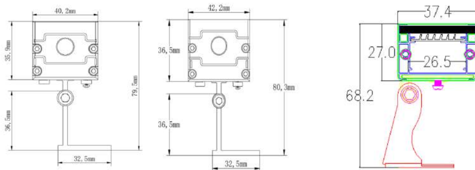
■产品尺寸图
