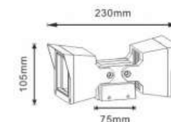
■产品尺寸图
