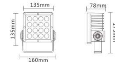
产品尺寸图
