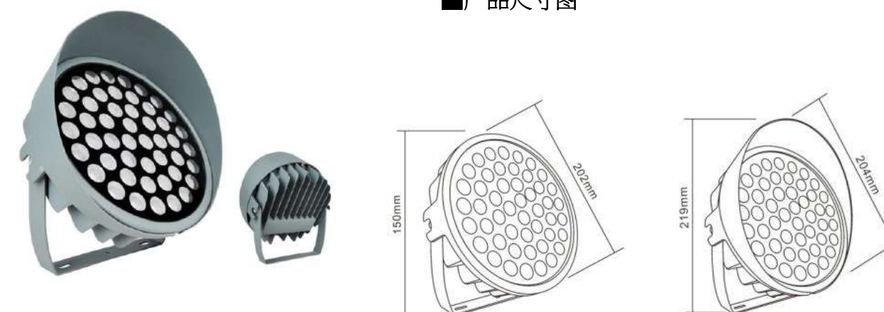
产品尺寸图
