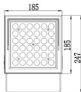
■产品尺寸图
