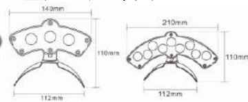
产品尺寸图
