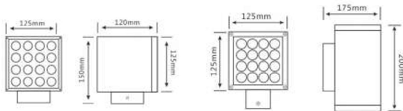
产品尺寸图
