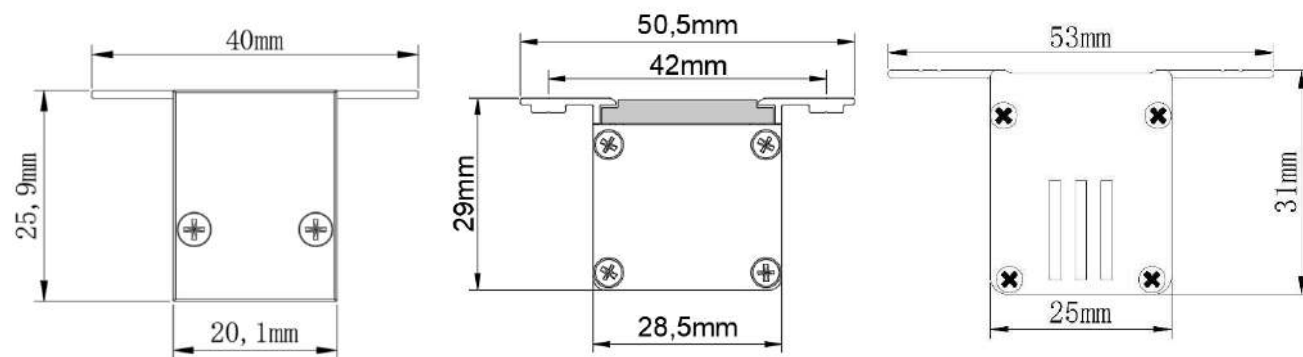
产品尺寸图
