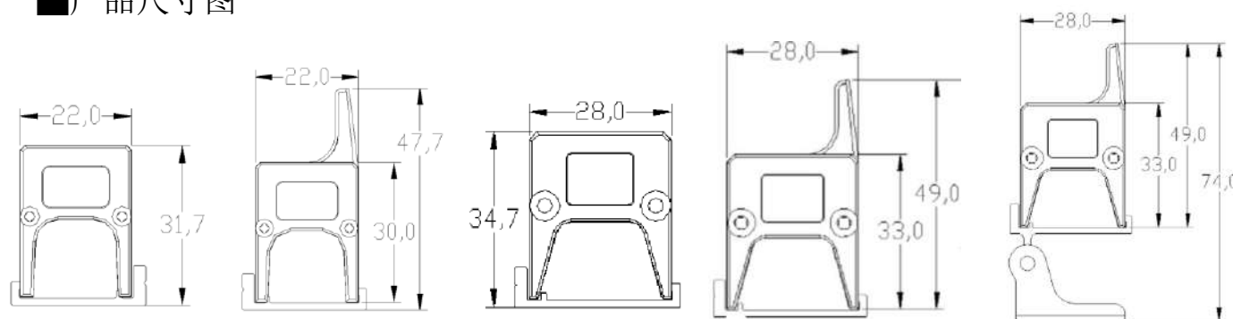
产品尺寸图
