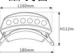
产品尺寸图
