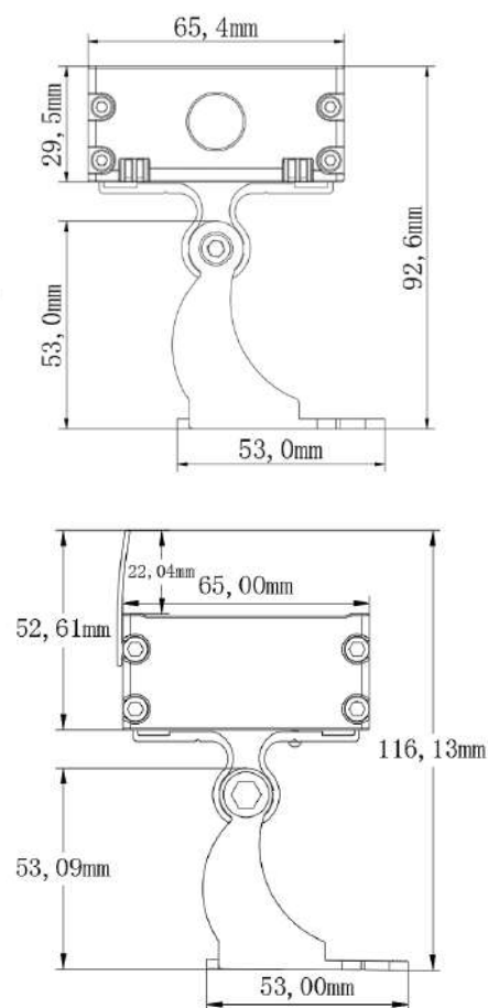
产品尺寸图
