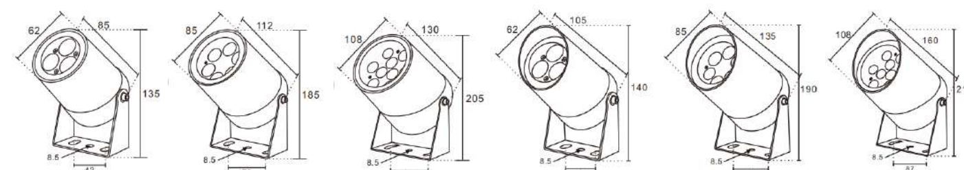
■产品尺寸图
