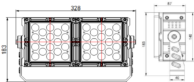
产品尺寸图
